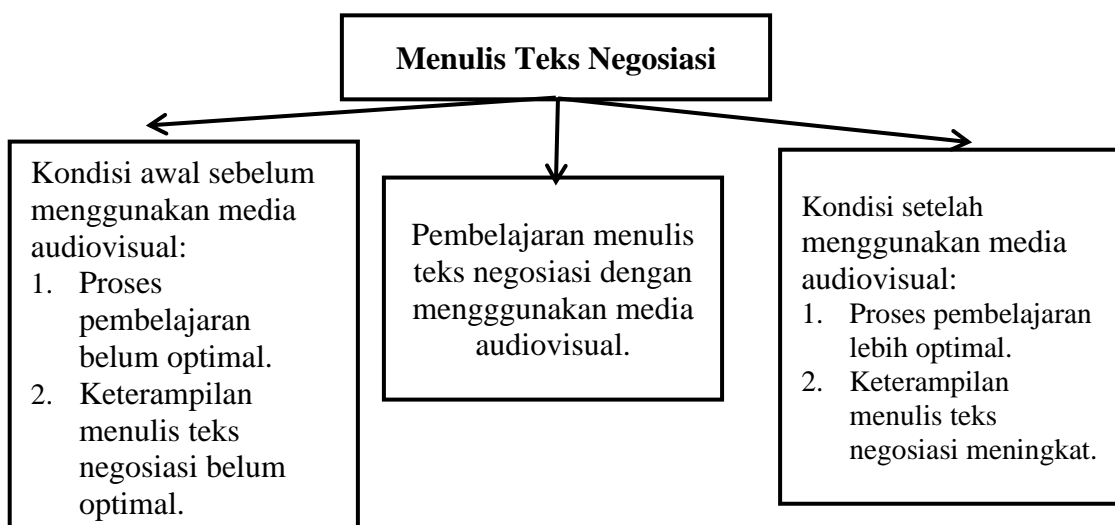
Gambar 1.1. Kerangka Berfikir
